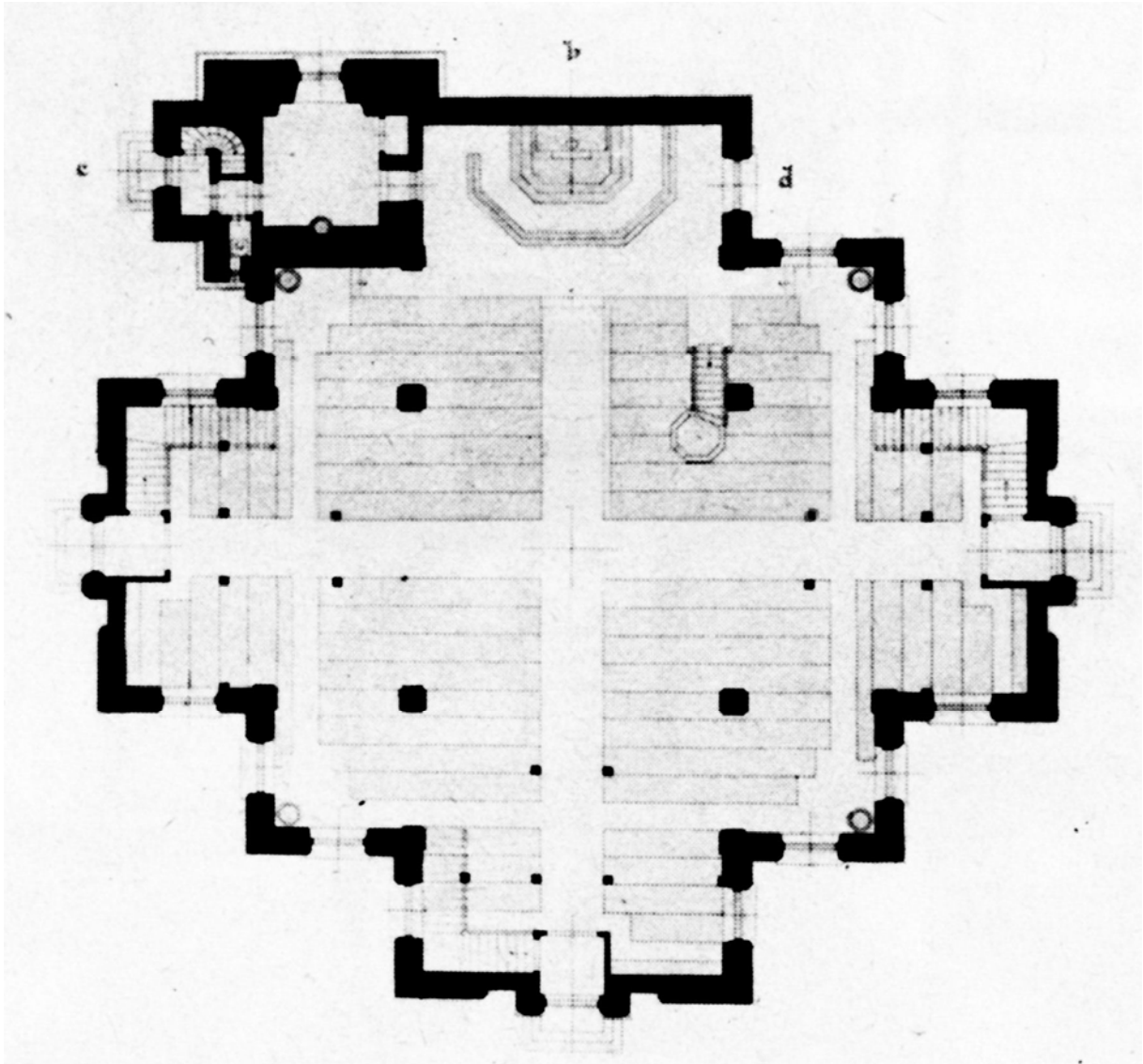
Kuolemajärven uuden kirkon pohjapiirros
